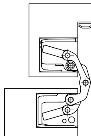
Blokkozijn 180°
