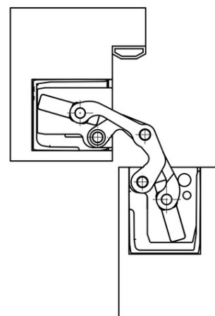
Blokkozijn 90°
